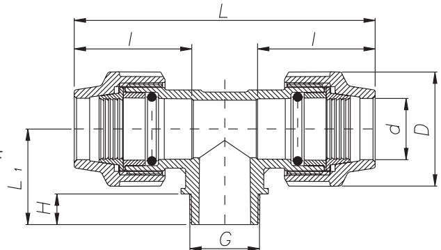
TI A 90° CON DERIVAZIONE MASCHIO 90° TEE WITH THREADED MALE TAKE OFF
